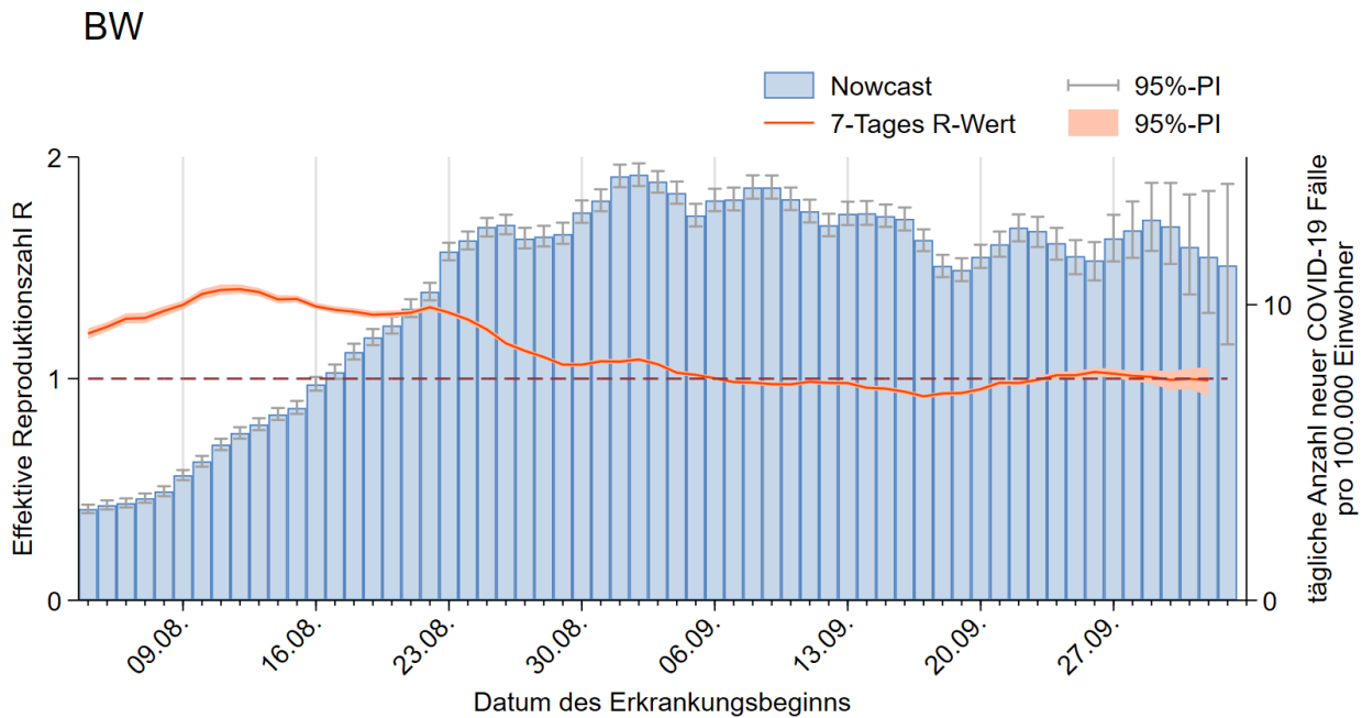
Abbildung 16: Schätzung des Verlaufs der Anzahl der COVID-19-Erkrankungsfälle (Nowcast) und des 7-Tages R-Wertes (effektive Reproduktionszahl) mit 95%-Prädiktionsintervall (95%-PI) in Baden-Württemberg; RKI Datenstand: 07.10.2021.
