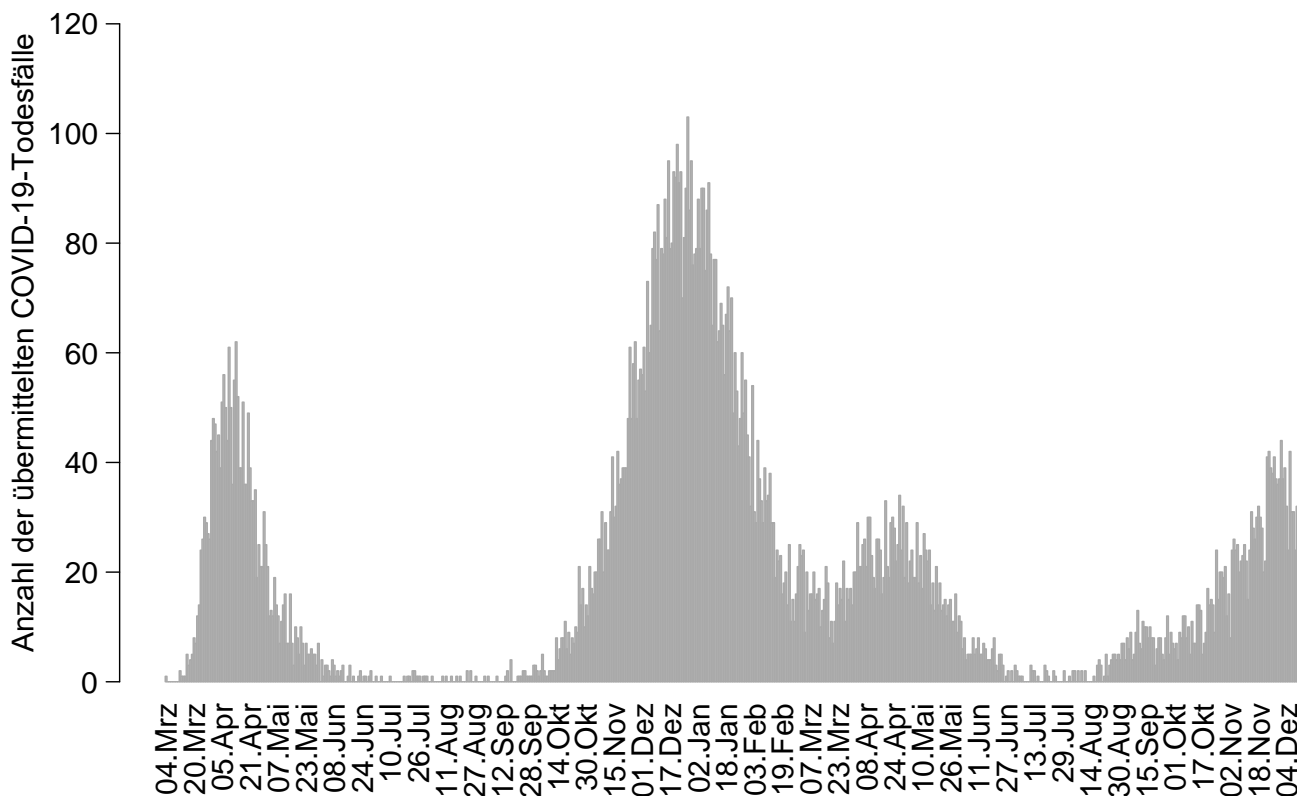
Abbildung 4: Anzahl der übermittelten Fälle, die mit und an COVID-19 verstorben sind, nach Sterbedatum, Baden-Württemberg, Stand: 14.12.2021, 16:00 Uhr.
